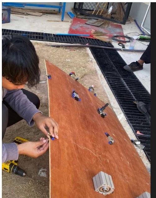
ภาพที่ 7 ขั้นตอนการยึดตัวและกระบอกสูบนิวมेटิกส์
