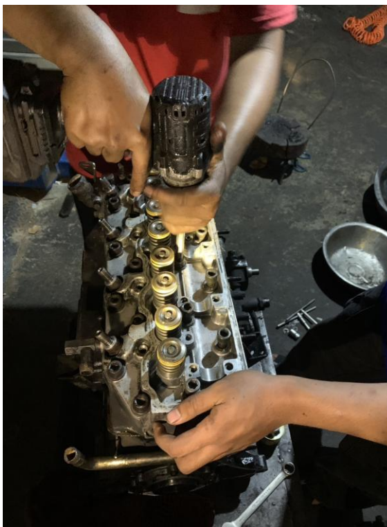
รูปภาพที่ 4.20 ตั้งมอค ตั้งวาล์ว
