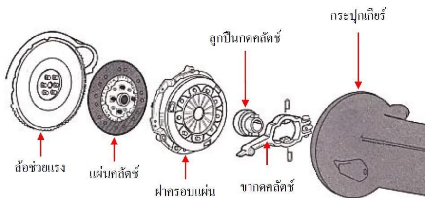
ภาพแสดงลักษณะของชุดคลัตช์
