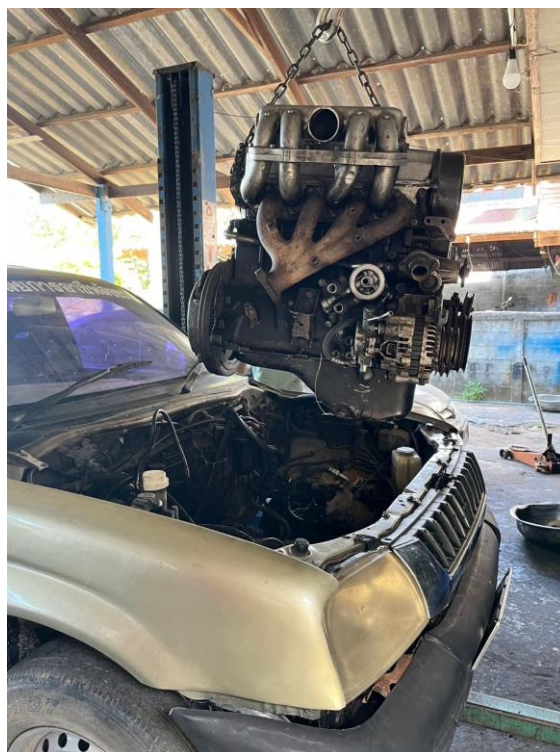
รูปภาพที่ 4.23 ยกเครื่องใส่บอดี้รถ
