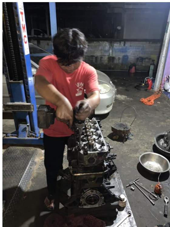
รูปภาพที่ 4.19 ปิดฝาหัว
