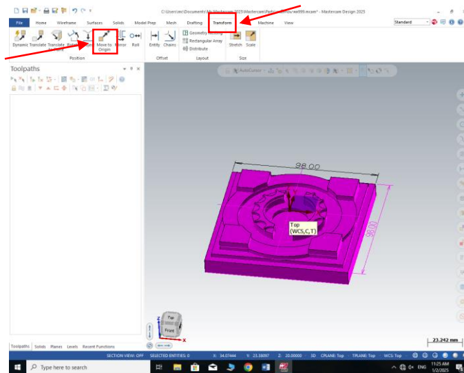
ภาพการดำเนินงานรูปภาพที่ 3 การกำหนดจุดศูนย์ขึ้นงานขึ้นมาด้านบน ( ที่มา : นายองศา เลิศงาม และคณะ, 2567 )
