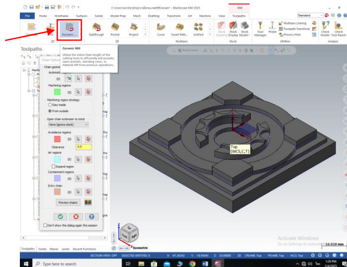
ภาพการดำเนินงานรูปภาพที่ 6 คลิกเข้าไปที่โหมด Dynamic Mill เพื่อทำการสร้างเส้นทางการตัด เฉือน ( ที่มา : นายองศา เลิศงาม และคณะ, 2567 )
