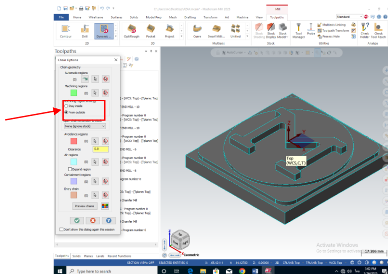
รูปภาพที่ 3.19 เลือก From outside เพื่อทำการตัดเฉือนชิ้นงานจากด้านนอก ในกรณีที่ต้องการตัดเฉือนชิ้นงานจากด้านในให้เลือก Stay inside ( ที่มา : นายองศา เลิศงาม และคณะ, 2567 )
