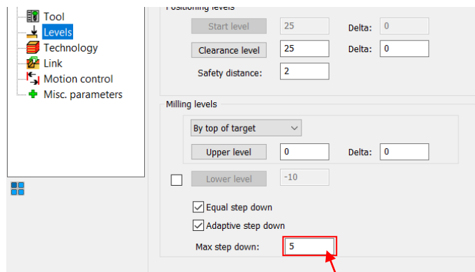
ภาพที่ 19 ภาคผนวก ก. ใส่ค่าการกัดลงมาในแต่ละครั้ง (ที่มา : นายยมนา สาสศรี และคณะ,2567)
