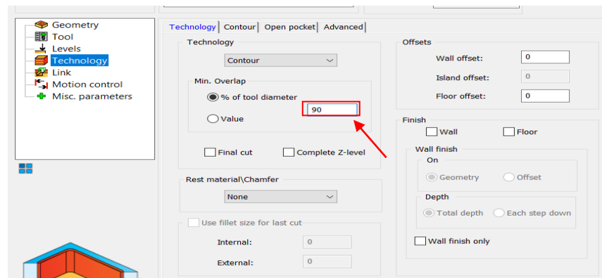
ภาพที่ 3.23 ในหมวด Technology ทำการตั้งค่าเปอร์เซ็นต์ไม่ให้เกิดกััดโดนขึ้นงานมากเกินไป (ที่มา : นายยมนาธ สารศรี และคณะ,2567)
