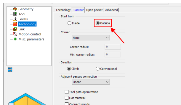
ภาพที่ 3.24 ในหมวด Contour ให้เลือกคำว่า Outside เพื่อกัดขึ้นงานจากด้านนอกเข้ามา (ที่มา : นายยมนาธ สารศรี และคณะ,2567)
