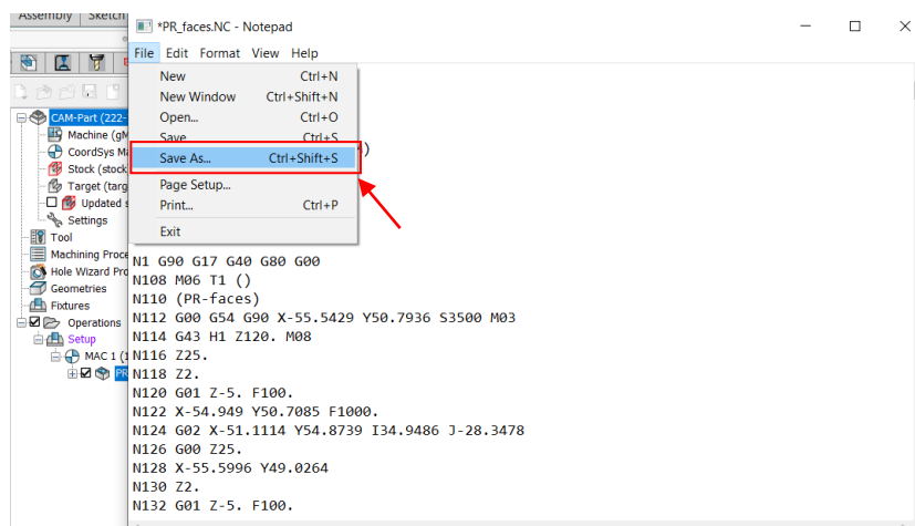
ภาพที่ 3.28 ทำการ Save G-code เพื่อนำไปเข้าเครื่อง CNC ต่อไป (ที่มา : นายยมนาท สารศรี และคณะ,2567)
