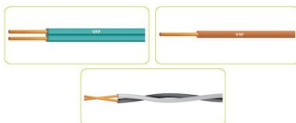
รูปภาพที่ 2.6 แสดงสาย ไฟฟ้าชนิดอ่อน (Flexible Wire)
