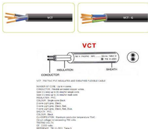
รูปภาพที่ 2.5 แสดงสาย ไฟฟ้าชนิดอ่อน (Flexible Wire)
