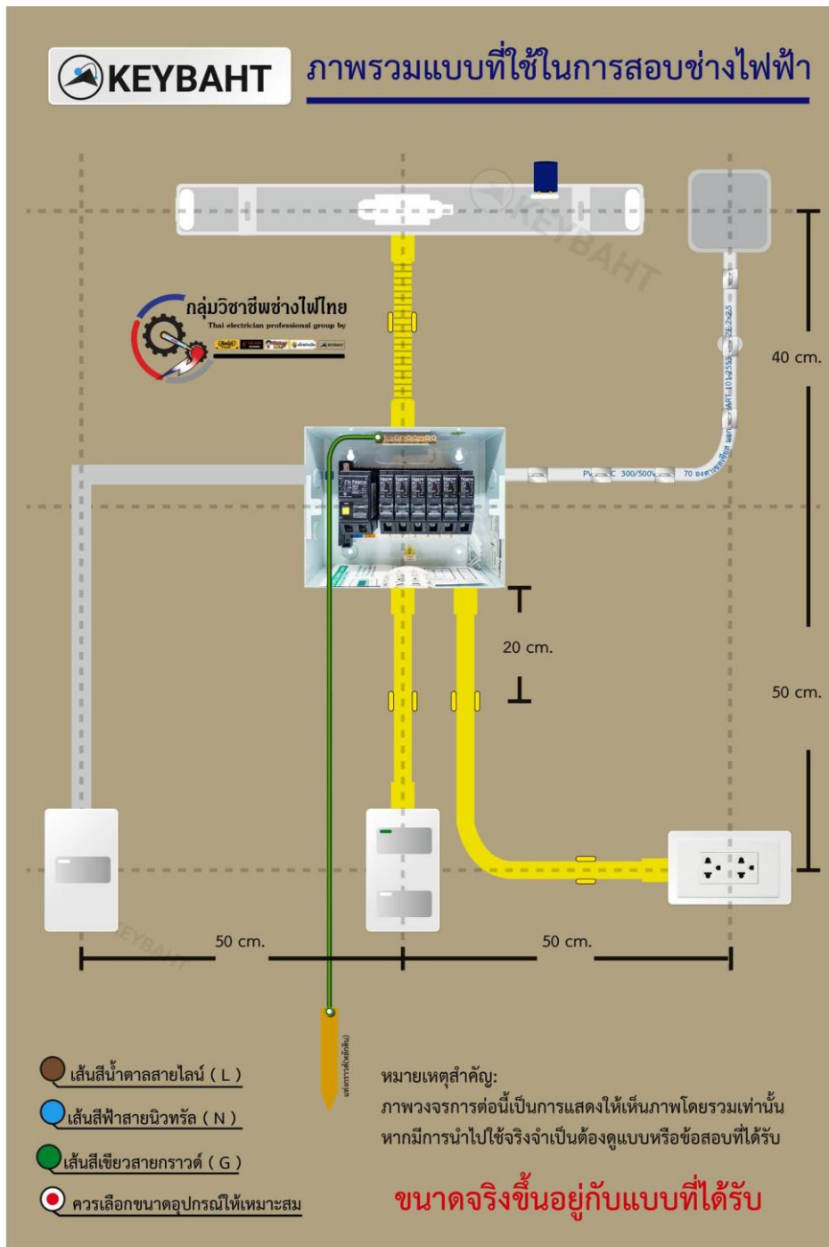
รูปภาพที่ 1 แสดงแบบมาตรฐานของกรมฝีมือแรงงาน
