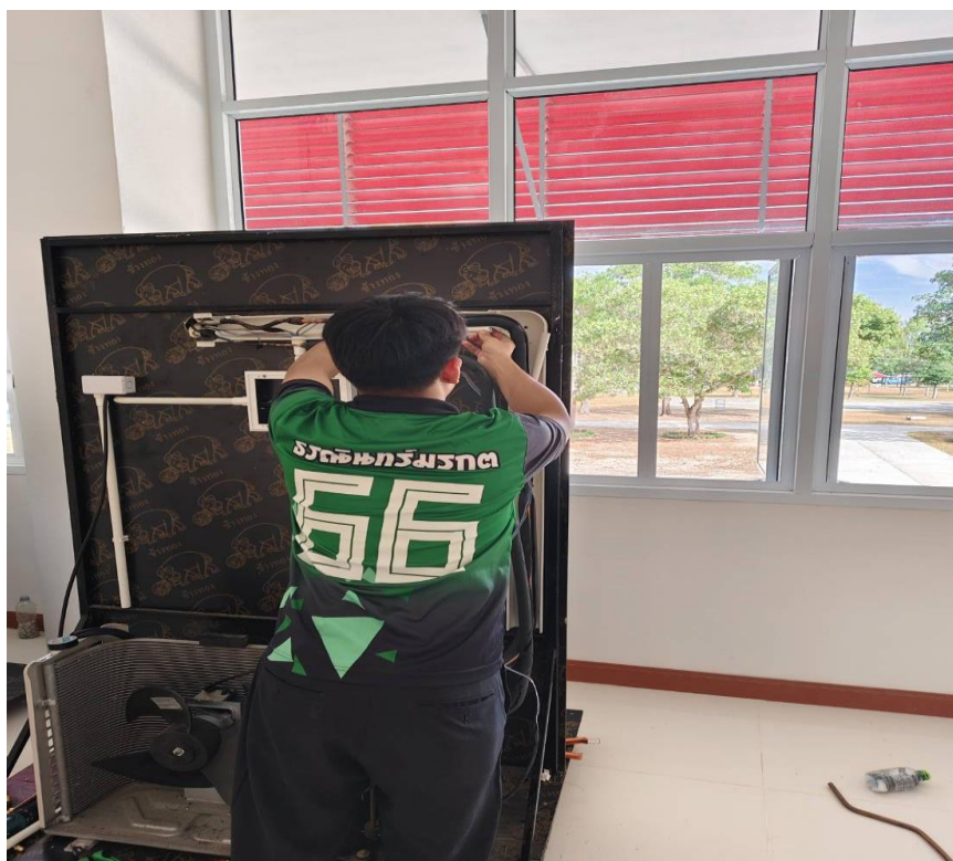
รูปภาพที่ 12 แสดงการเดินท่อและสายไฟชุดส่วนประกอบแอร์ด้านหลัง
