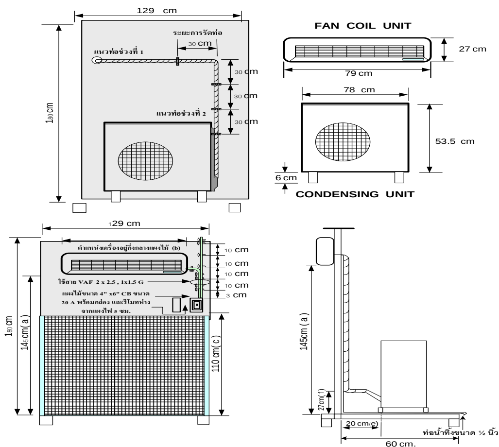
แบบชุดฝึกการติดตั้งเครื่องปรับอากาศแบบแยกส่วน
